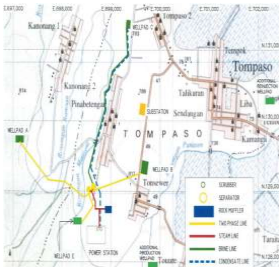
Layout pembangunan Lahendong 5 dan 6 Sumber: project appraisal document
