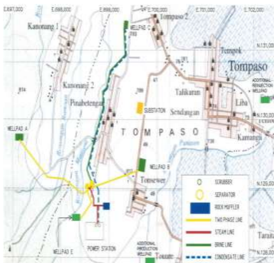
Layout pembangunan Lahendong 5&6 Sumber: project appraisal document
