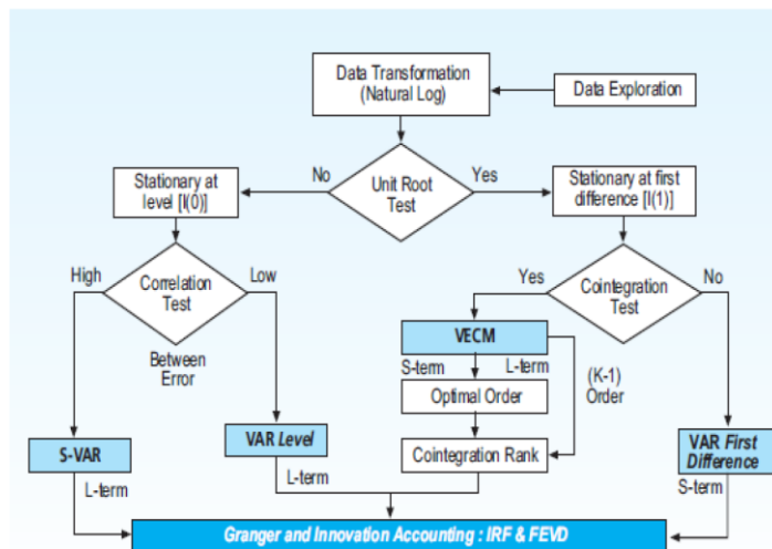
Gambar 4 Tahapan Analisis VAR
